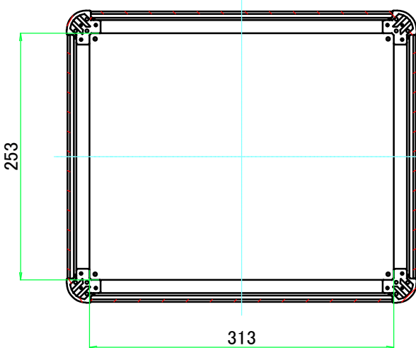
C-C ( 1 : 5.5 )
